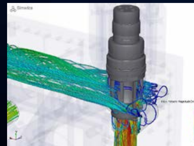
Einströmung in das Servocartridge-Ventil (X700)
